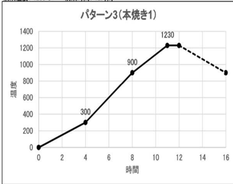
[パターン3 (本焼き1)] 焼成温度: 1230°C 焼成時間: 12時間
